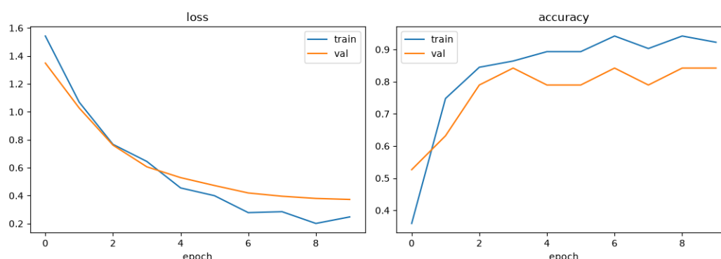
איור 4. עקומות אימון (הפסד ודיוק, אימון מול val) עבור מודל 70/30 Extended.
