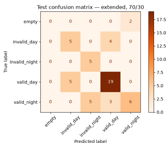
איור 5. מטריצת בלבול למבחן, מודל 70/30 Extended.
