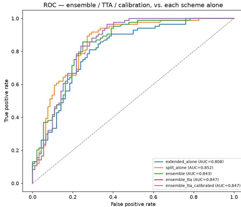
איור 7. עקמות ROC — וריאציות שילוב/TTA/כיוול מול כל מודל לבדו.
