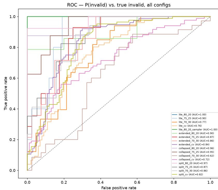
איור 6. עקמות ROC, כל 17 הקונפיגורציות הבודדות.
